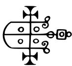
GAAP
